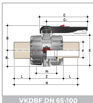
VKDBF DN 65-100
