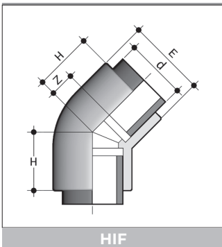
HIF
