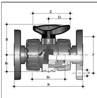
VKDOF DN 15-50
