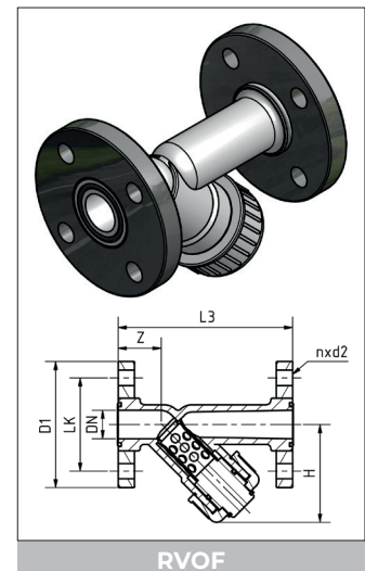
RVOF
