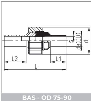
BAS - OD 75-90
