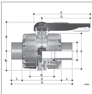
VKDDF DN 65-100
