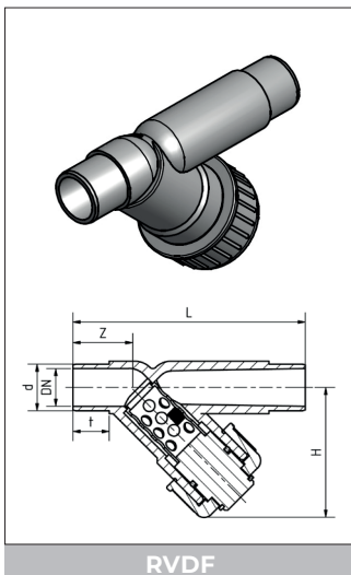
RVDF
