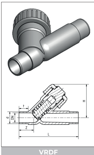
VRDF
